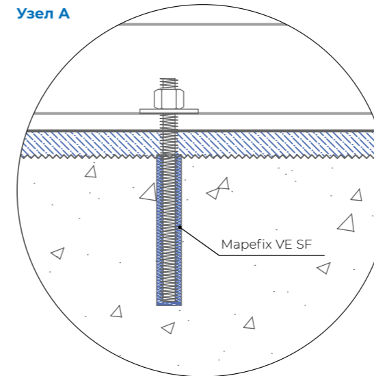
Узел А
