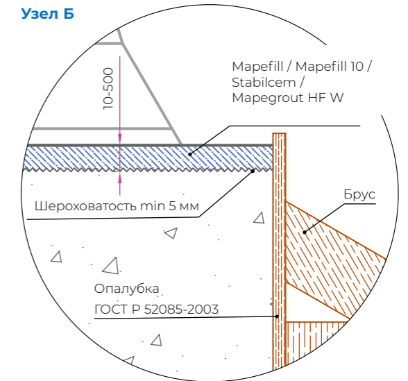
Узел Б
