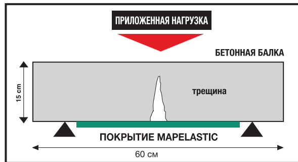
Рисунок 1. Защита волосистой трещины с помощью Mapelastic на нижней грани бетонной балки, подверженной изгибающей нагрузке
