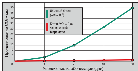
Рисунок 2. Защита пористого бетона с помощью Mapelastic от ускоренной карбонизации (30% CO 2 )
