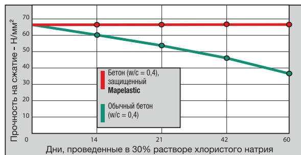
Рисунок 4. Защита бетона с помощью Mapelastic от снижения механической прочности, вызываемого воздействием антиобледенительных солей
