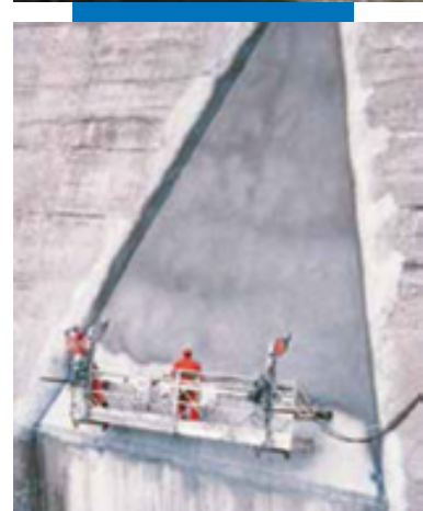
Нанесение Mapelastick на дамбу распылением
