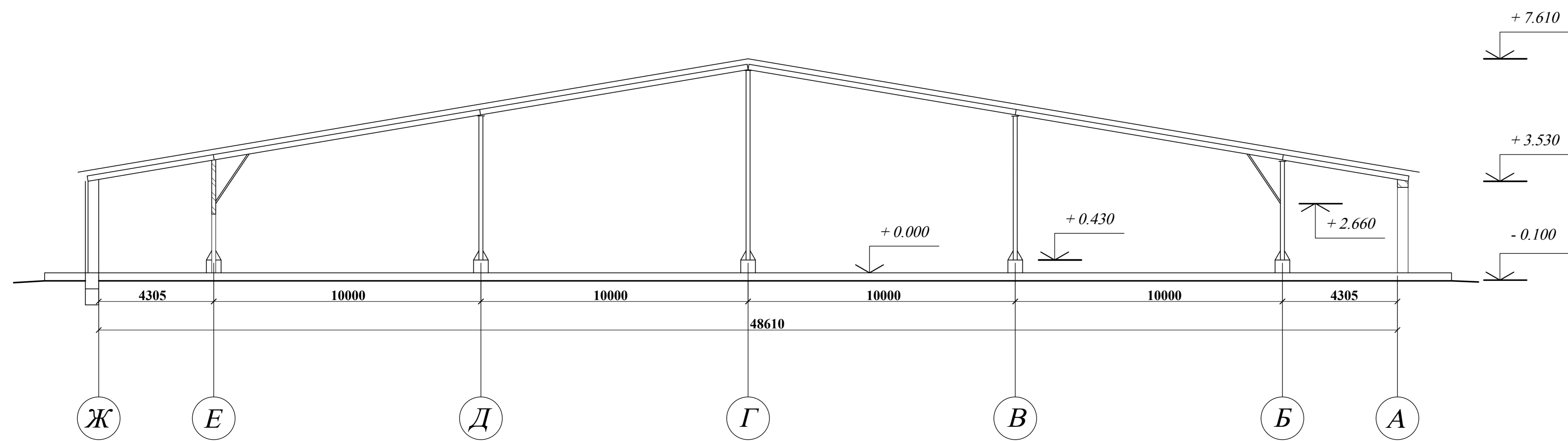
Рисунок П.4.6 – Разрез 1-1
